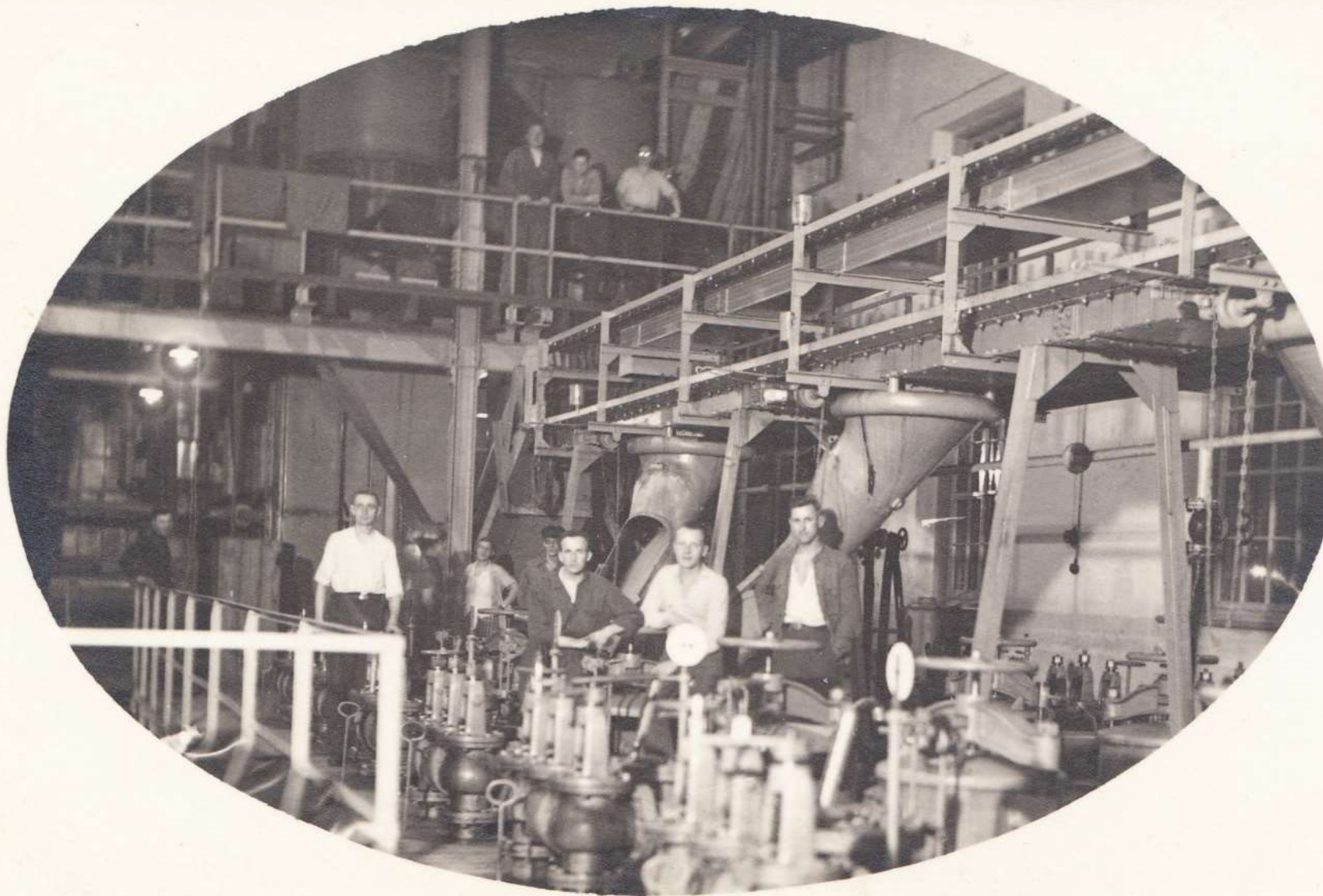
Centrifūgu stacijas, kur žāvēja un tīrīja cukuru.
