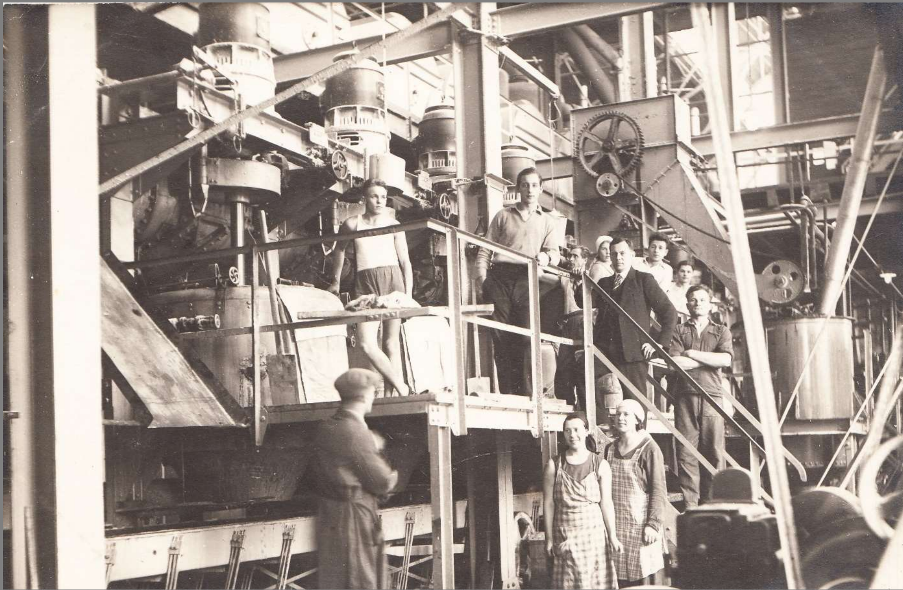
Centrifūga, kurā atdala šķidro frakciju no kristāla (melasi no cukura).
